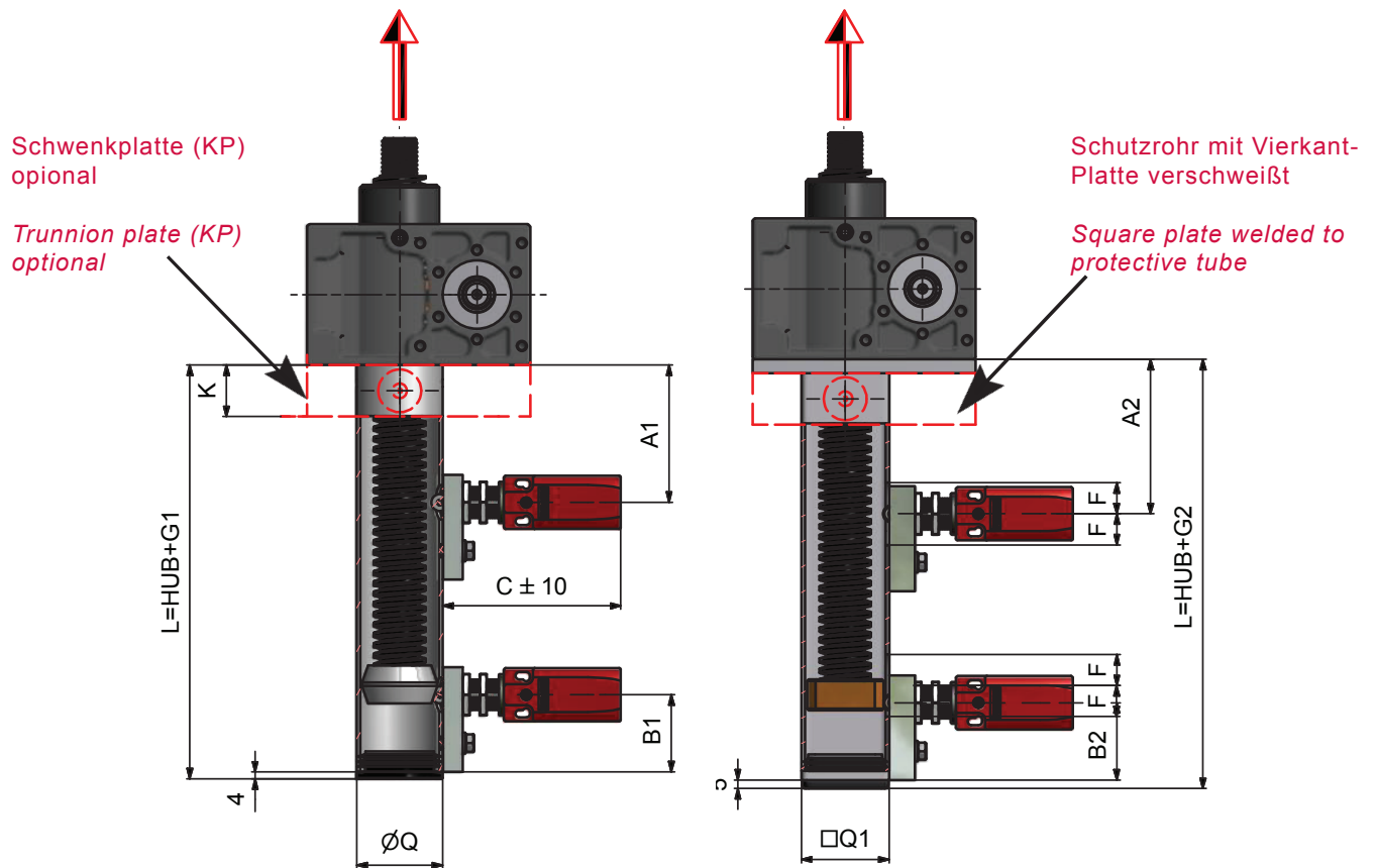
Endschalteranbau variabel Limit switch assembly adjustable
